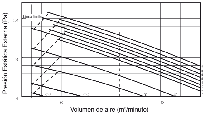
Diagrama P-Q
