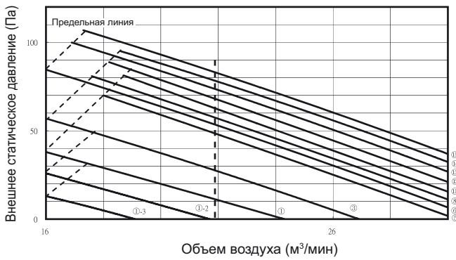
График P-Q
