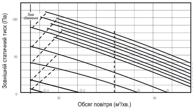
Графік P-Q
