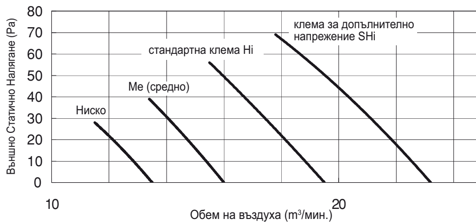
S-45PN1E5, S-50PN1E5 P-Q КРИВА
