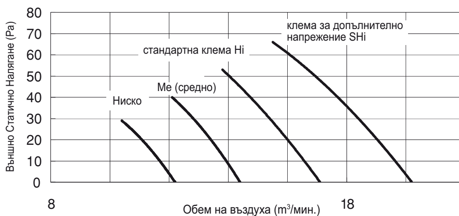
S-36PN1E5 P-Q КРИВА
