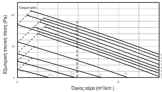
Διάγραμμα P-Q
