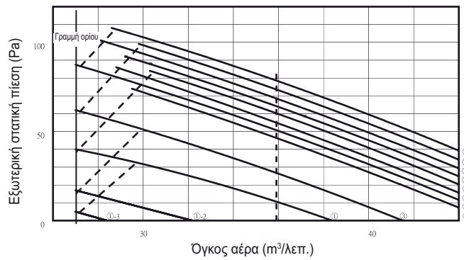
Διάγραμμα P-Q
