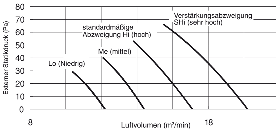
S-36PN1E5 P-Q-KURVE
