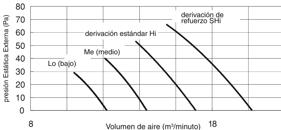
S-36PN1E5 Curva P-Q
