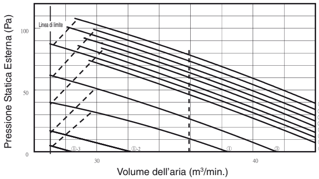
Disegno P-Q
