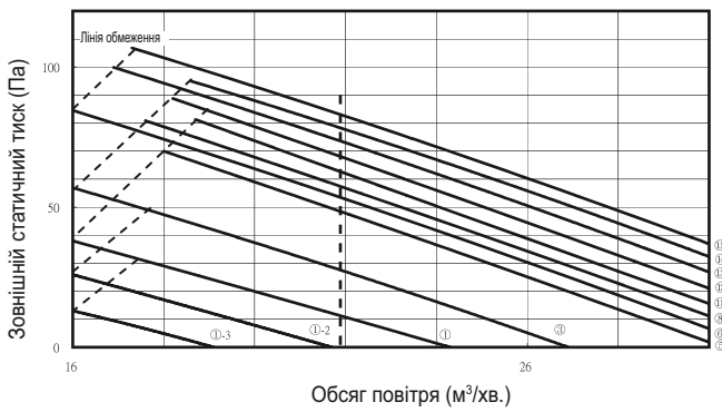
Графік P-Q
