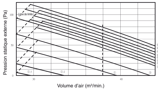
Schéma P-Q
