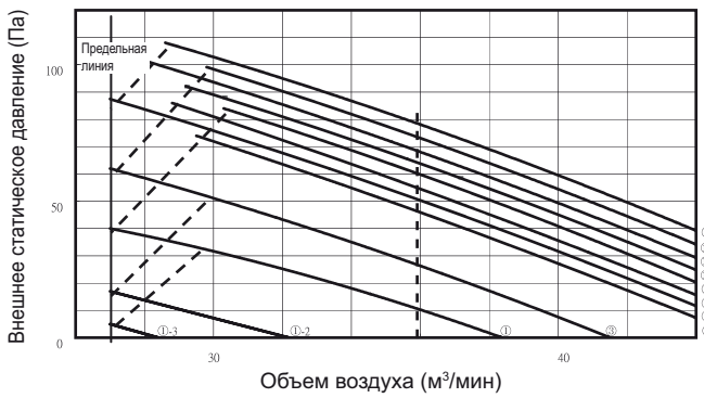
График P-Q
