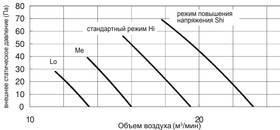
S-45PN1E5, S-50PN1E5 КРИВАЯ P-Q
