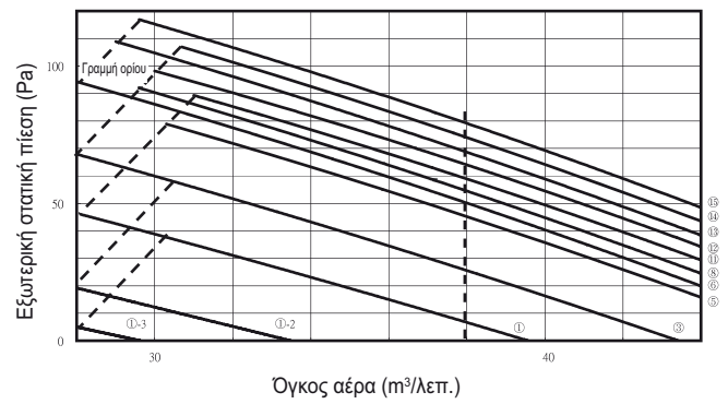
Διάγραμμα P-Q
