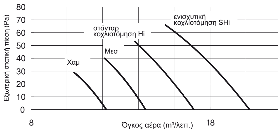
S-36PN1E5 ΚΑΜΠΥΛΗ P-Q
