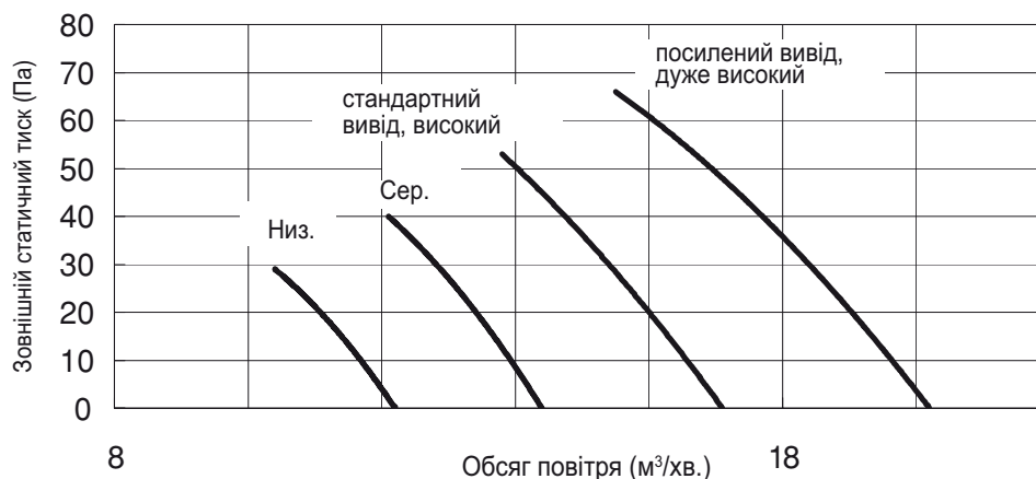
S-36PN1E5 КРИВА P-Q
