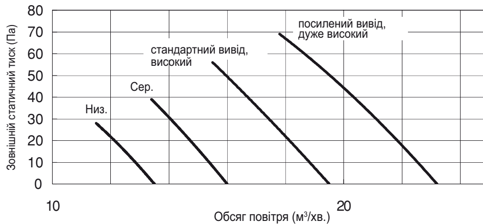
S-45PN1E5, S-50PN1E5 КРИВА P-Q
