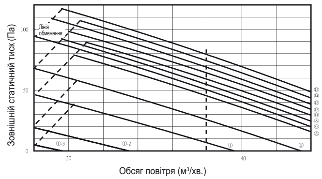
Графік P-Q
