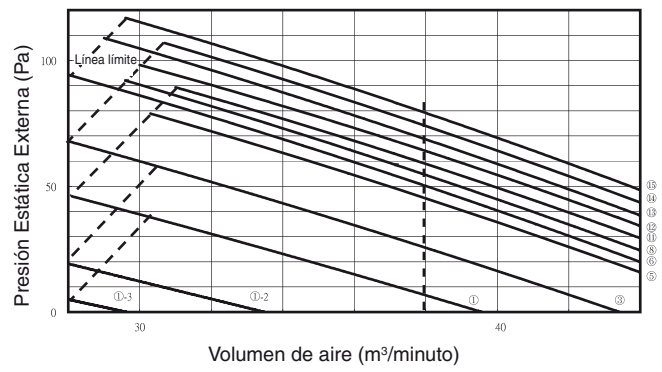
Diagrama P-Q
