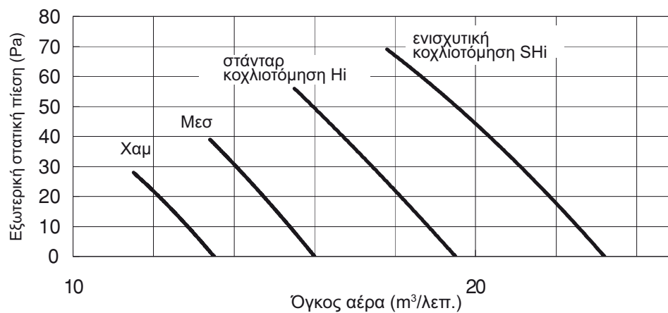
S-45PN1E5, S-50PN1E5 ΚΑΜΠΥΛΗ P-Q
