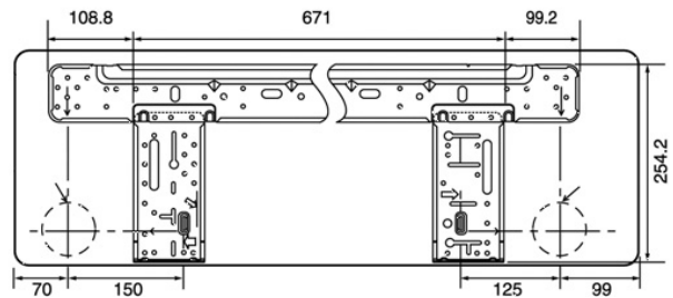
Montageplatte
