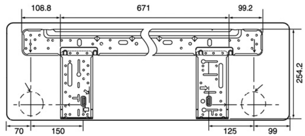
Montageplatte
