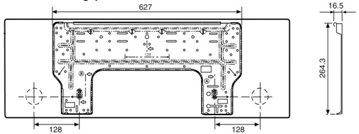
Montageplatte
