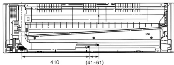
Rückansicht
