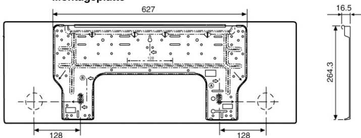
Montageplatte
