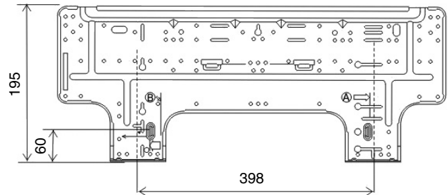
Montageplatte
