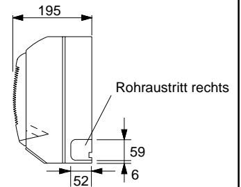
Seitenansicht
