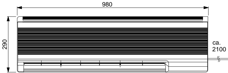
Frontansicht
