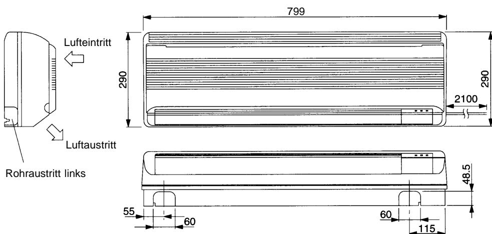
Frontansicht
