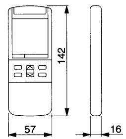
Drahtlose Fernbedienung
