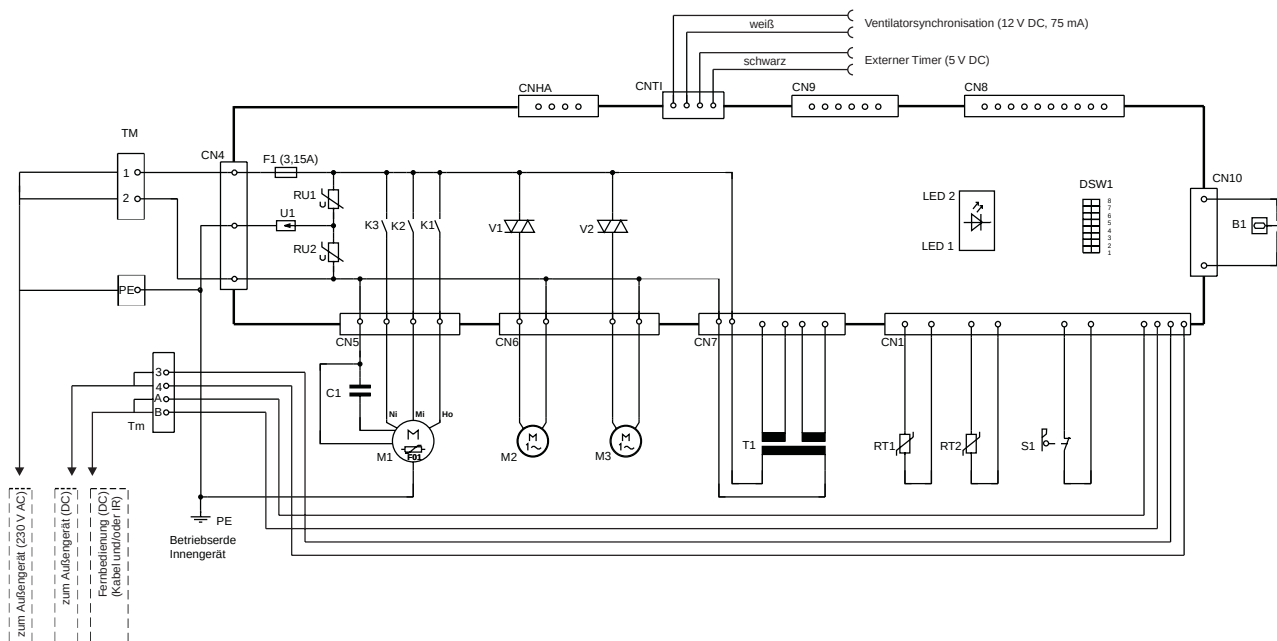
Innengerät (CS-P112U1JP)
