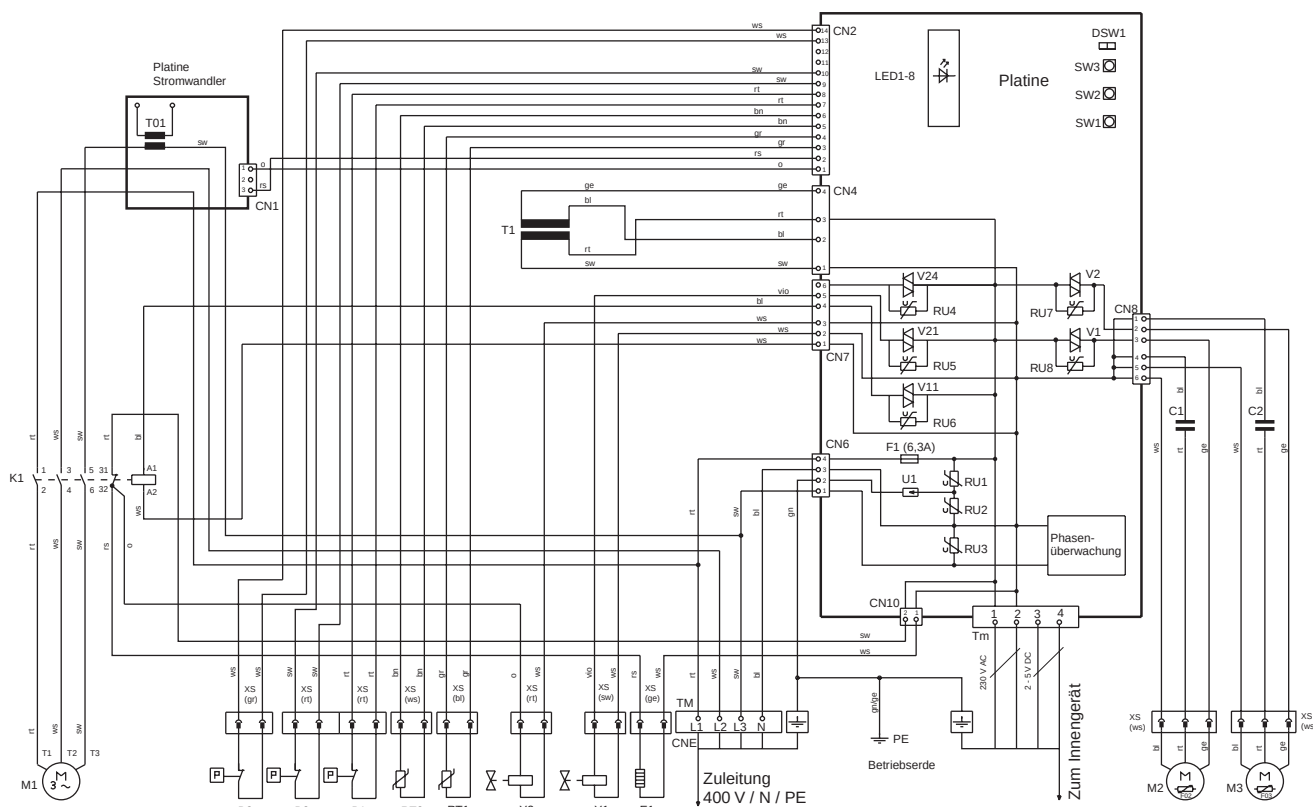
Außengerät (CU-P112H1XP)
