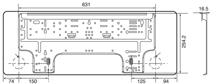
Montageplatte
