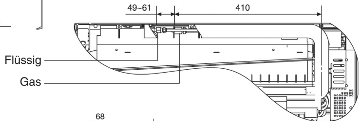
Rückansicht
