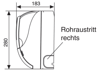
Seitenansicht
