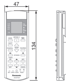
Drahtlose Fernbedienung
