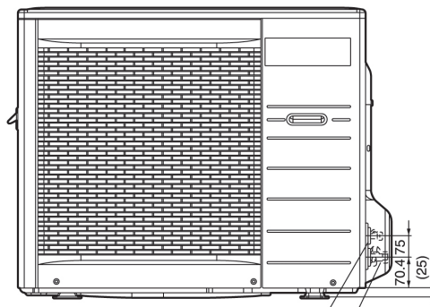
Frontansicht
