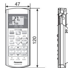
Drahtlose Fernbedienung
