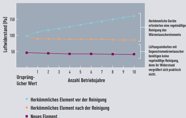
Verlauf des Luftwiderstands in Abhängigkeit von der Anzahl der Betriebsjahre
