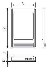
Hotel-Fernbedienung (CZ-REZC2) Fernsensor (CZ-CSRC2)
