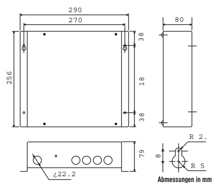
Kommunikationsadapter (CZ-CFUNC2)
