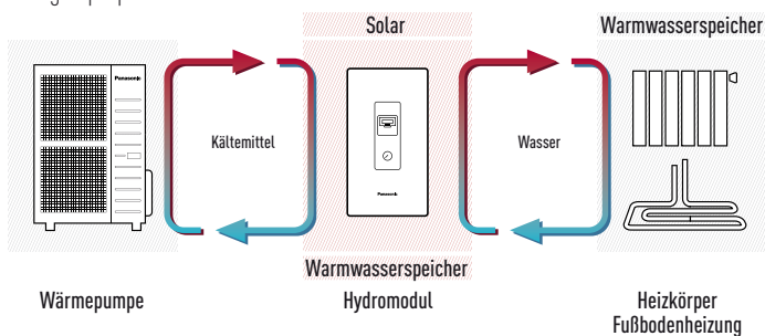
Beispiel eines Splitsystems
