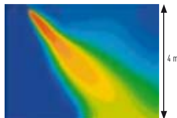
Komfortverbesserung durch die Luftführung
