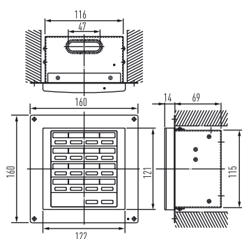
Schalt-/Statusafel (CZ-ANC2)
