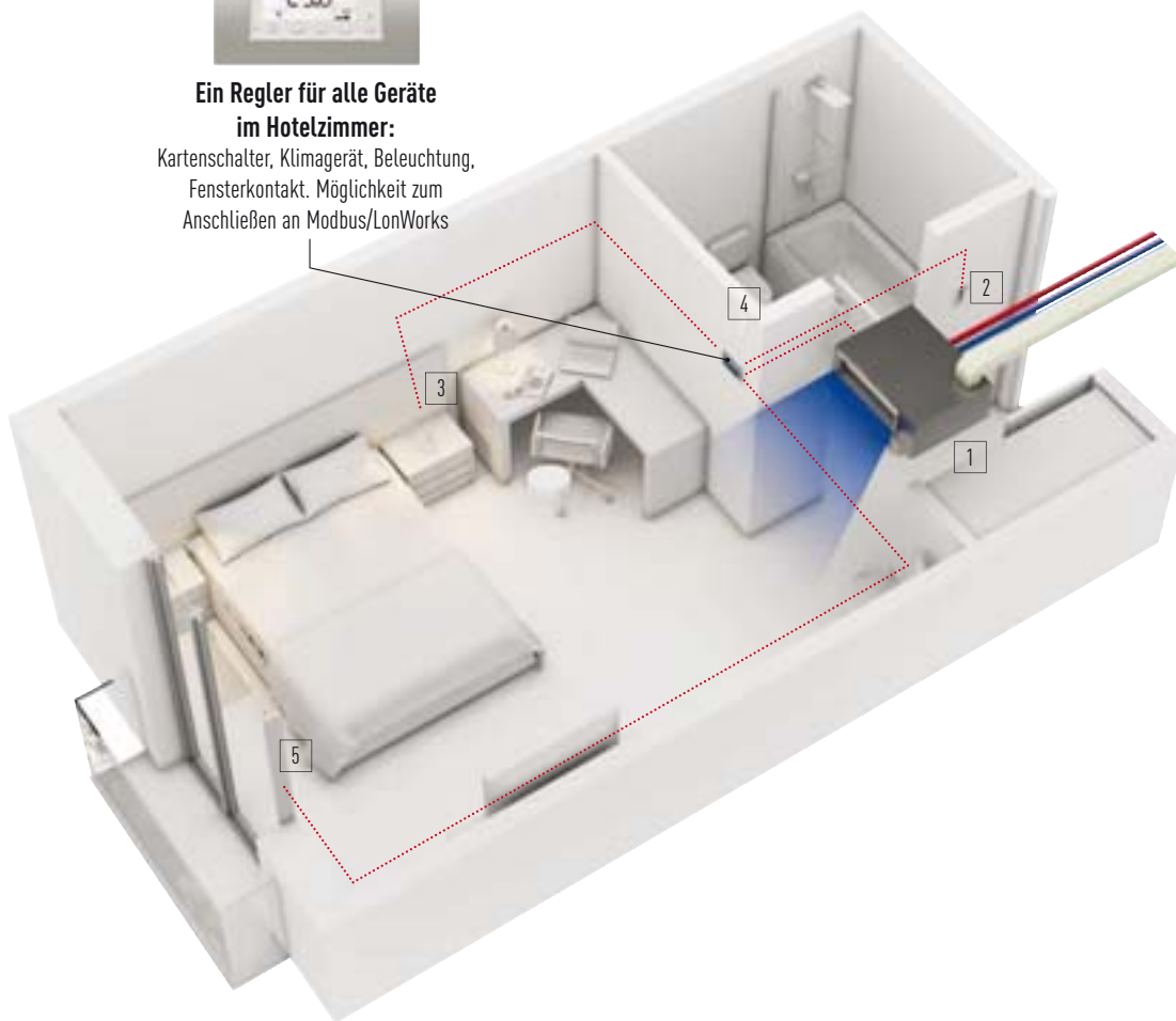
1 Innengerät: Kanalgeräte mit mittlerer Pressung
