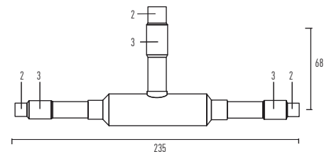
Flüssigkeitsleitung
