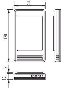
Fernsensor (CZ-CSRC3)
