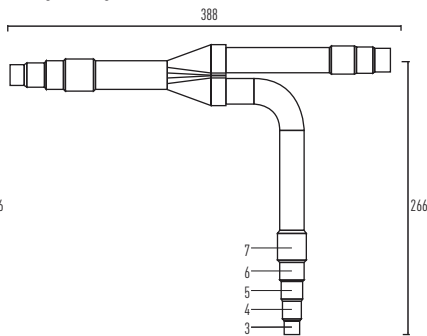
Heißgasleitung
