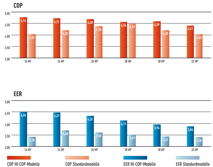
Bester COP der Branche (Modelle mit HI-COP-Modus bei Volllast)
