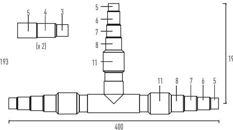
Heißgasleitung
