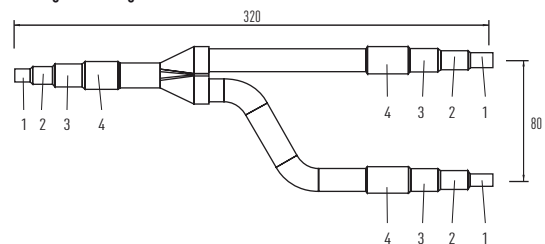
Flüssigkeitsleitung
