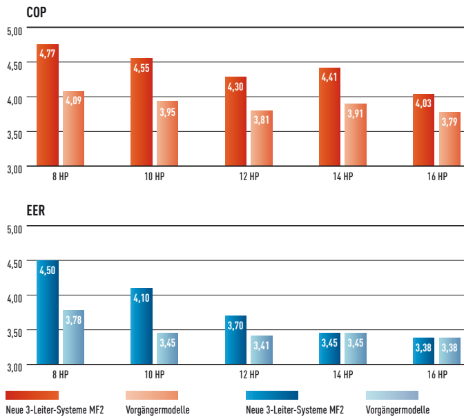
Bester COP der Branche (Standardmodelle bei Volllast)
