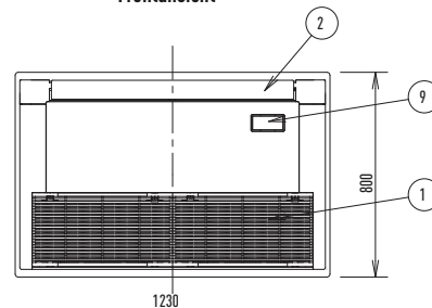
Frontansicht
