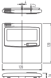
Design-Kabel-Fernbedienung (CZ-RTC5)
