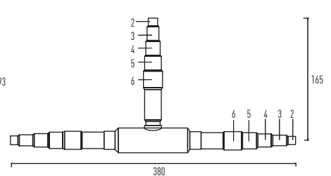
Flüssigkeitsleitung
