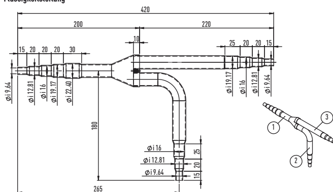
Flüssigkeitsleitung
