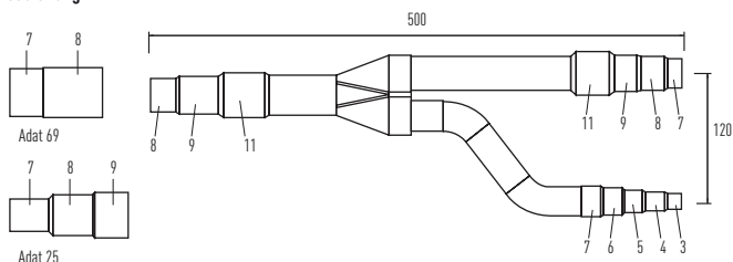
Gasleitung
