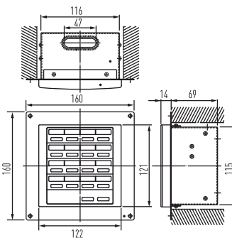
Schalt-/Statustafel (CZ-ANC2)
