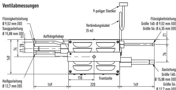
WRG-Box-Steuereinheit* In Kombination mit CZ-P56HR3 bzw. CZ-P160HR3 immer erforderlich. * CZ-CAPE2 (für alle Innengeräte außer Wandgeräte) CZ-CAPEK2 (für Wandgeräte)
