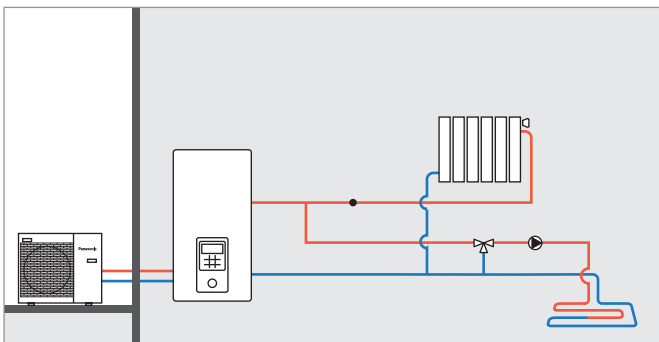
Zwei Heizkreise mit Aquarea Splitsystem H-Generation, ohne Pufferspeicher
