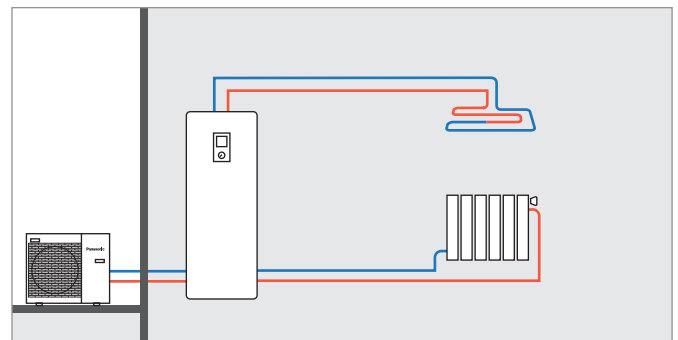
Zwei Heizkreise mit Aquarea Kombi-Hydromodul H-Generation Ausführung „B“, ohne Pufferspeicher
