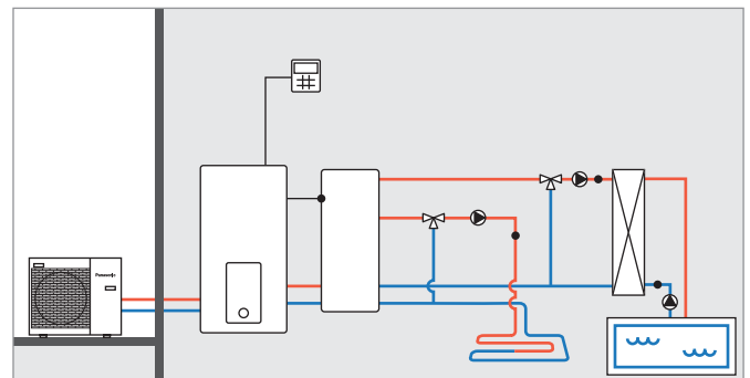
Zwei Heizkreise mit Aquarea Splitsystem H-Generation, Pufferspeicher und Schwimmbadheizung
