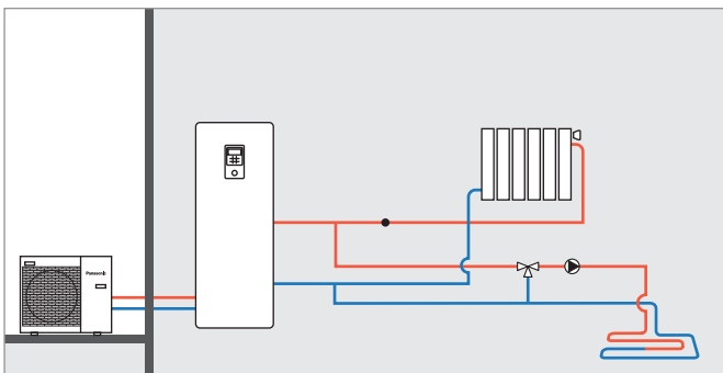
Zwei Heizkreise mit Aquarea Kombi-Hydromodul H-Generation, ohne Pufferspeicher
