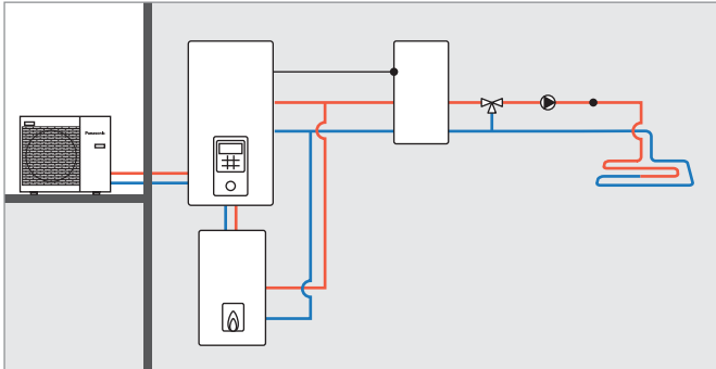
Bivalentes Heizungssystem mit Aquarea Splitsystem H-Generation, Pufferspeicher und Mischventil
